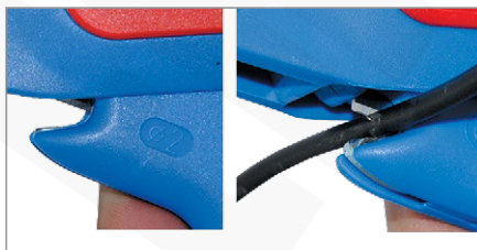
Odcięcie przewodu
