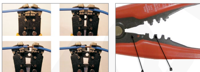
Zdejmowanie izolacji
