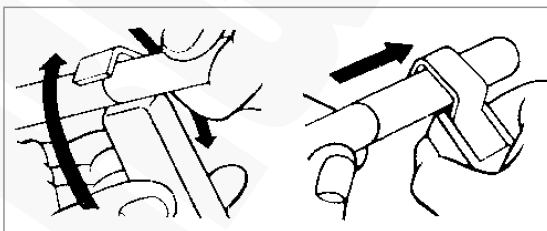
Zdejmowanie izolacji z „końca” kabla
