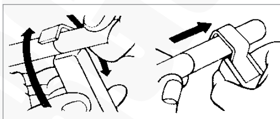
Zdejmowanie izolacji z „konca” kabla
