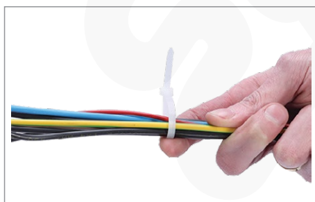
1.1 - Ręczne zaciąganie opasek kablowych - włożyć końcówkę opaski kablowej w jej zamek
