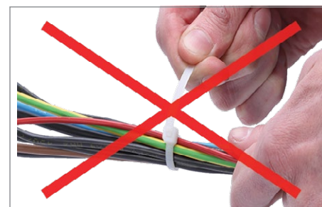
1.3 - Unikać przeginalnia opaski, nie poprawi to siły mocowania a może uszkodzić opaskę
